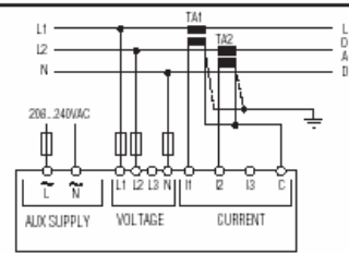
Двухфазное подсоединение Параметр P.03 установлен в 2рh
