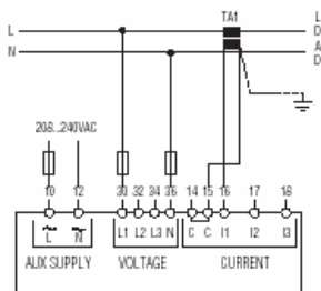
Однофазное подсоединение Параметр P.03 установлен в 1рh
