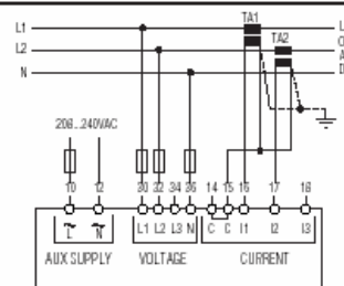
Двухфазное подсоединение Параметр P.03 установлен в 2рh
