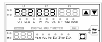
Установка усредненного фильтра (параметр P.02) в значение 3
